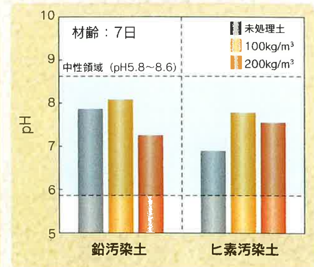
【pH 試験事例】
